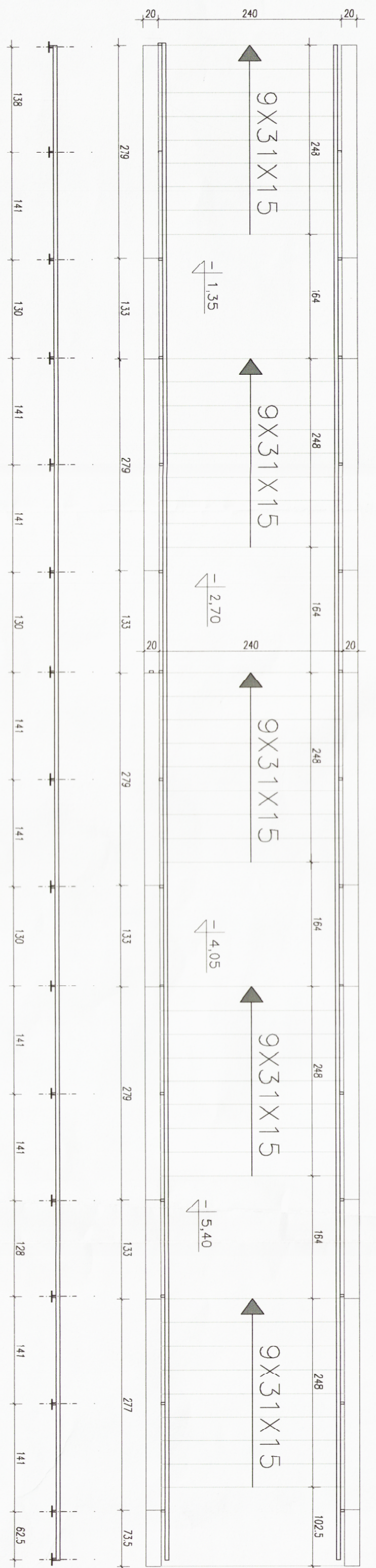
RZUT SCHODÓW
