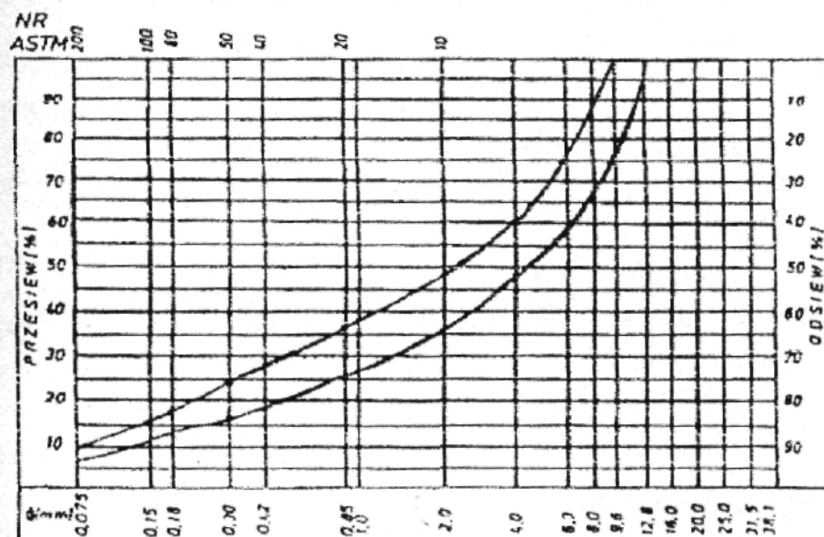
Rys. 4. Krzywe graniczne uziarnienia mieszanki mineralnej 0+12,5 mm do warstwy ścieralnej z betonu asfaltowego dla KR 3-6
