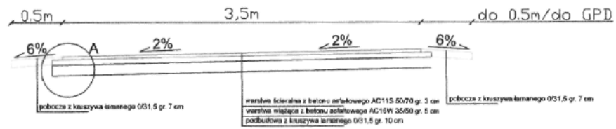
Przekrój poprzeczny drogi gminnej
