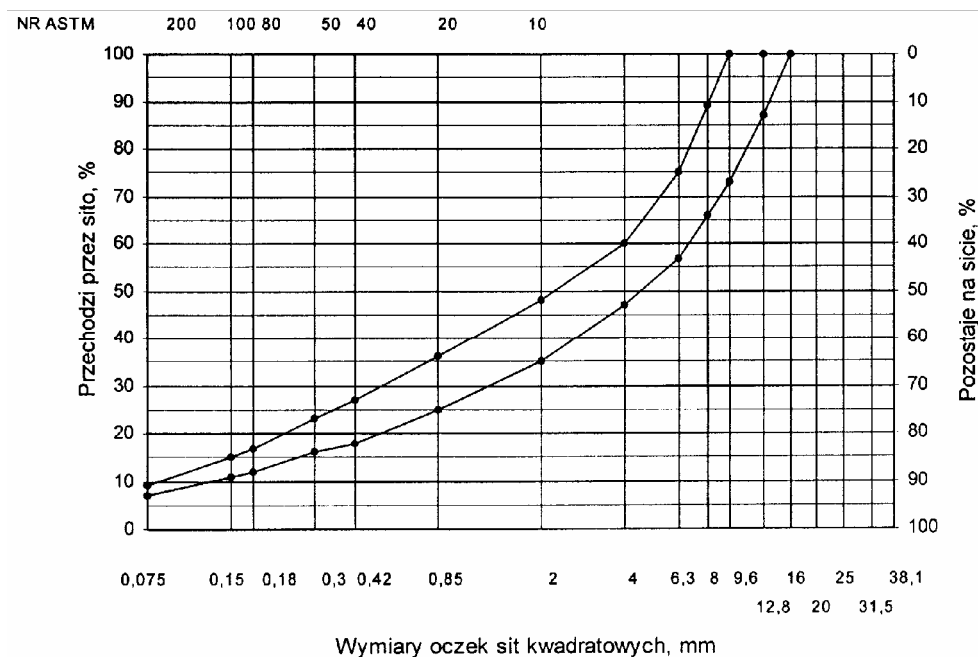
Rys. 1. Krzywe graniczne uziarnienia mieszanki mineralnej BA od 0 do 12,8 mm do warstwy ścieralnej nawierzchni drogi o obciążeniu ruchem od KR1 do KR2
